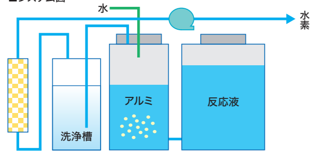
■システム図
